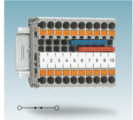
Durchgangsklemmen PT 2,5
