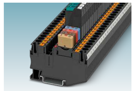
Thermische Schutzschalter für Überlast und Kurzschlusschutz
