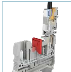
Reihenklemme ST 2,5/2P
