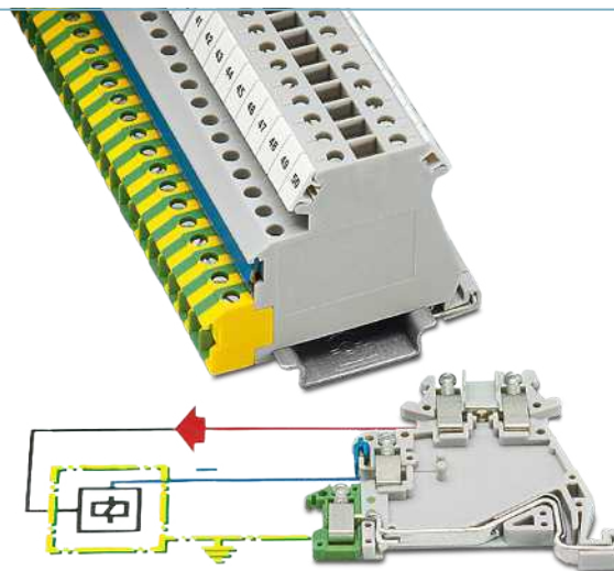
Sensor-/Aktor-Klemmen DOK 1,5
