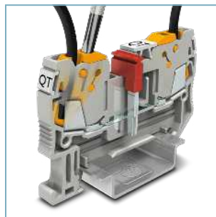
Reihenklemme QTC 2,5
