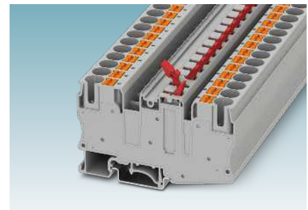
Hebel-Messertrennklemmen PT 10-MTL
