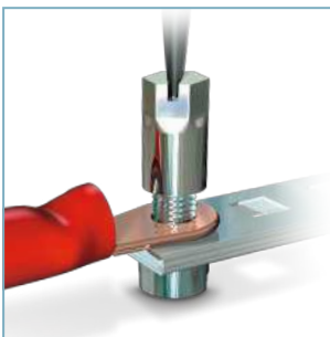
Klemmkörper einer Bolzenanschlussklemme
